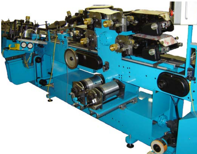
PRINTER MODULE
